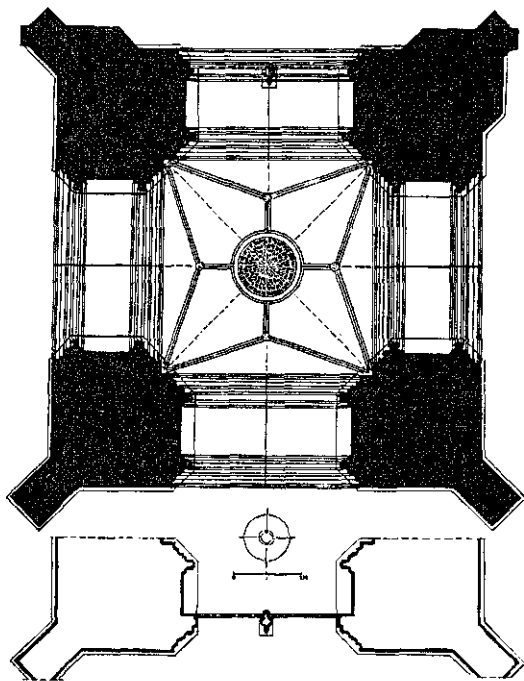
Onderste of eerste torenruimte
