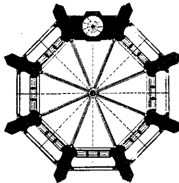
Lantaarn naar gewelf gezien
